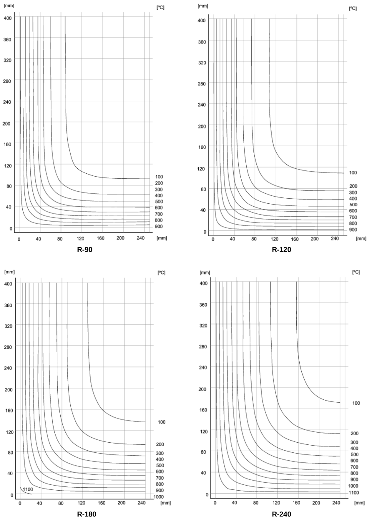
Figura C.5. Isothermas para cuartos de secci n de 800 x 500 mm expuestos por ambas caras
